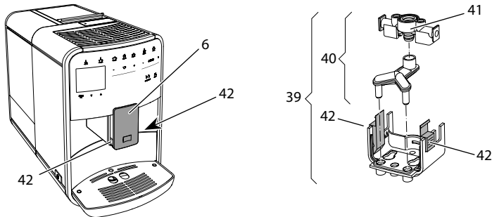
Abb. 24: Milcheinheit ausbauen
