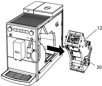
Kuva 16: Suodatusyksikön irrottaminen
