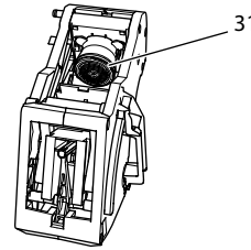
Şek. 17: Demleme ünitesinin temizlenmesi
