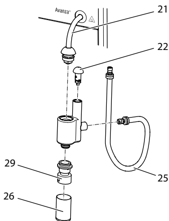
Obr. 15: Rozebání Cappuccinatore
