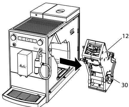
Joon. 16: Tõmbekambri väljavõtmine
