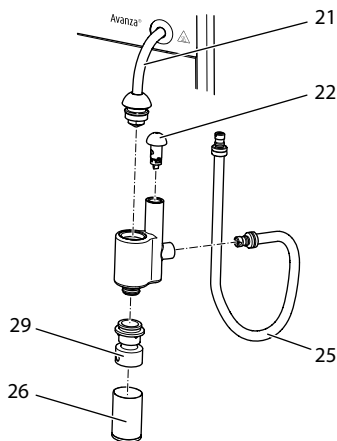
Рис. 15: Разборка капучинатора
