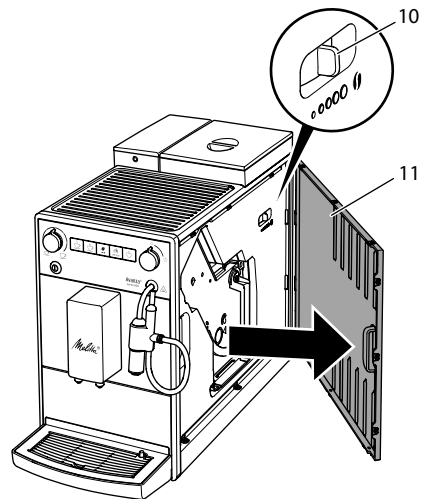
Afb. 14: Maalgraad instellen
