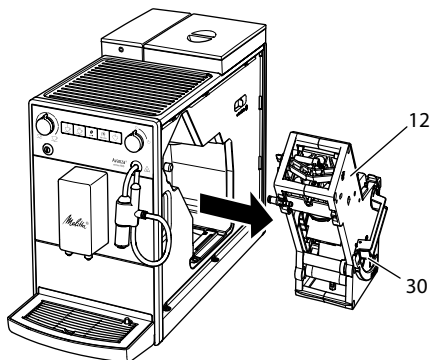
Obr. 16: Vymontovat spařovací jednotku
